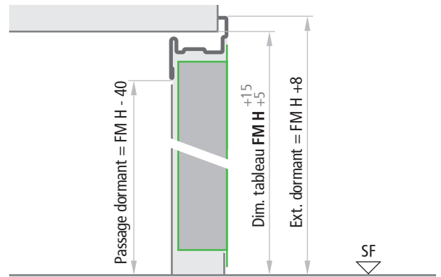
Porte sans battue inférieure - Coupe verticale
