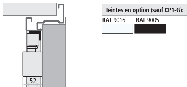
RC2-G PROGET (côté poussant)
